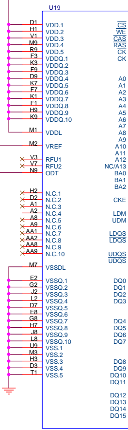
MT47H64M16HR-3:E
