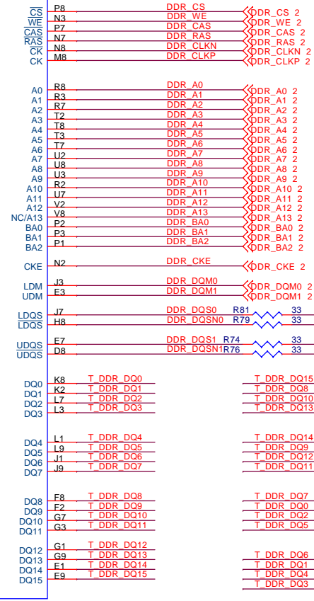
MT47H64M16HR-3:E
